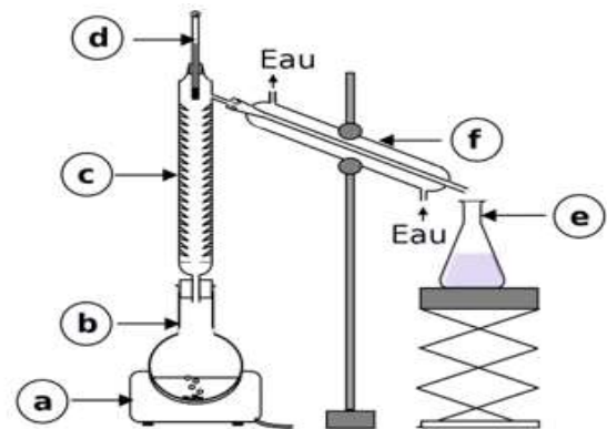
Dispositif de distillation fractionnée
